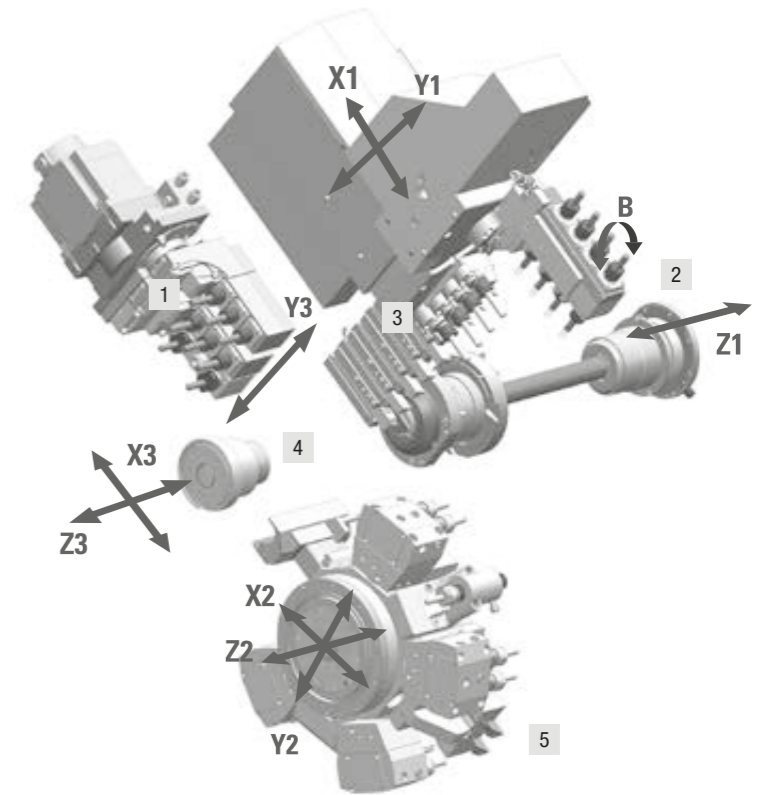
Typ VIII (Abbildung mit Option)
